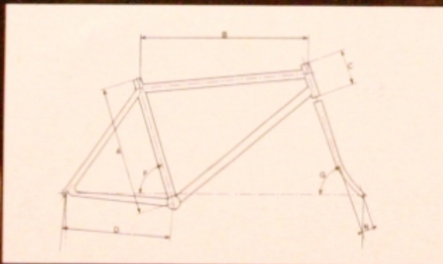
GEOMETRIE DES CADRES SUNN 26" TAILLES EN CM
