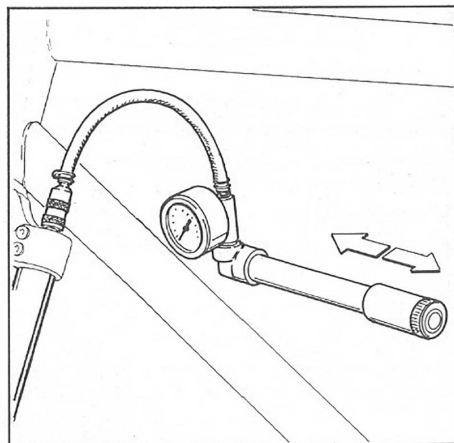
FIG. 6 Immettere aria dalla valvola, utilizzando la pompa speciale MARZOCCHI munita dello speciale ugello di gonfiaggio (rif. 103). Portare la pressione all'interno a circa 3,5 bar (psi 50). Riavvitare il cappuccio (303) di protezione. La pressione interna influenza il comportamento della forcella sia in fase di compressione che in quella di estensione. Ad una pressione più alta corrisponde una maggior durezza dell'azione ammortizzante. Per una regolazione corretta a seconda del tipo di utilizzo attenersi a quanto indicato sul foglio di istruzioni allegato.
