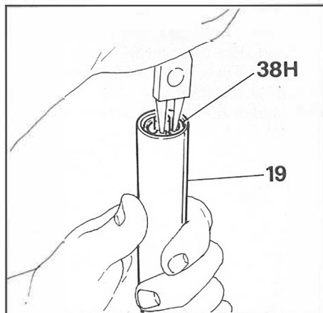
FIG. 5 Ingrassare l'anello OR' (4) e reinserire il tappo (17) con valvola montata dentro al tubo portante e spingerlo fino a superare l'alloggiamento dell'anello di fermo. Rimontare l'anello di fermo (38H) superiore.
